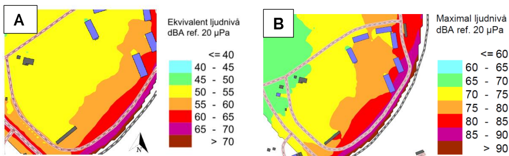
Figur 7: A redovisar ekvivalenta ljudnivåer från både väg och järnväg utan bulleråtgärder år 2040. B redovisar maximala ljudnivåer från bara järnvägen utan bulleråtgärder år 2040. Svart ring visar ungefärlig plats för planområde.
